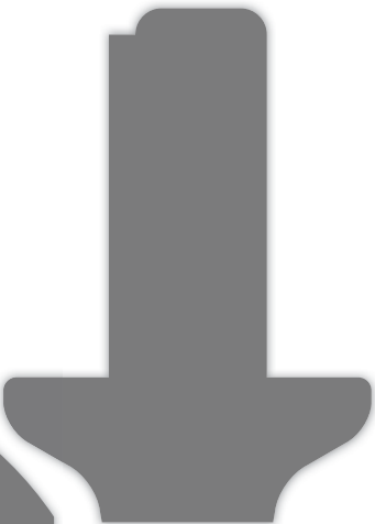
HWP7012 Astragal 2.437"x 1.750"
